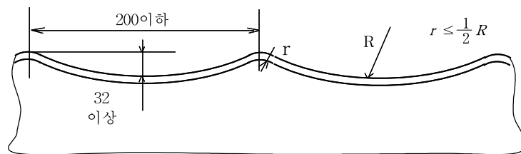
(b) 폭스형
