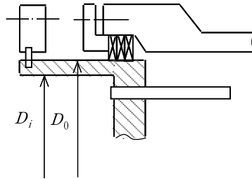
[그림 31.7] 유동두 그랜드형 관판
