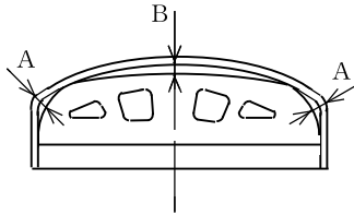
[그림 13.3] 경판 편차 계측방법
