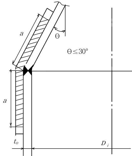
[그림 30.9] 보강링의 유효범위
