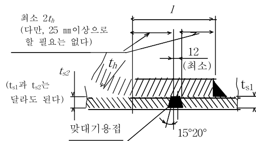
(f) 중간경판
