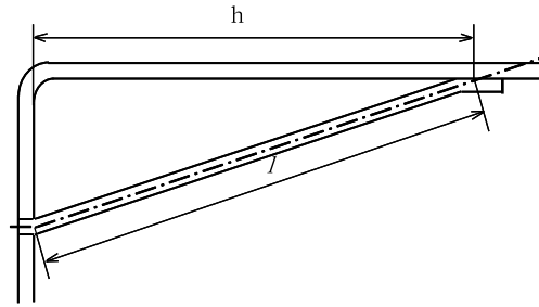
[그림 8.3] 경사스테이
