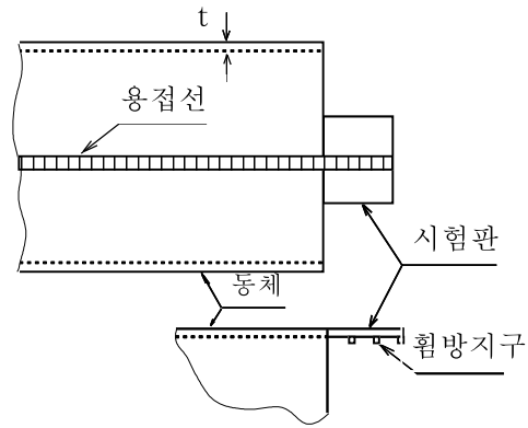
[그림 14.1] 시험판의 부착
